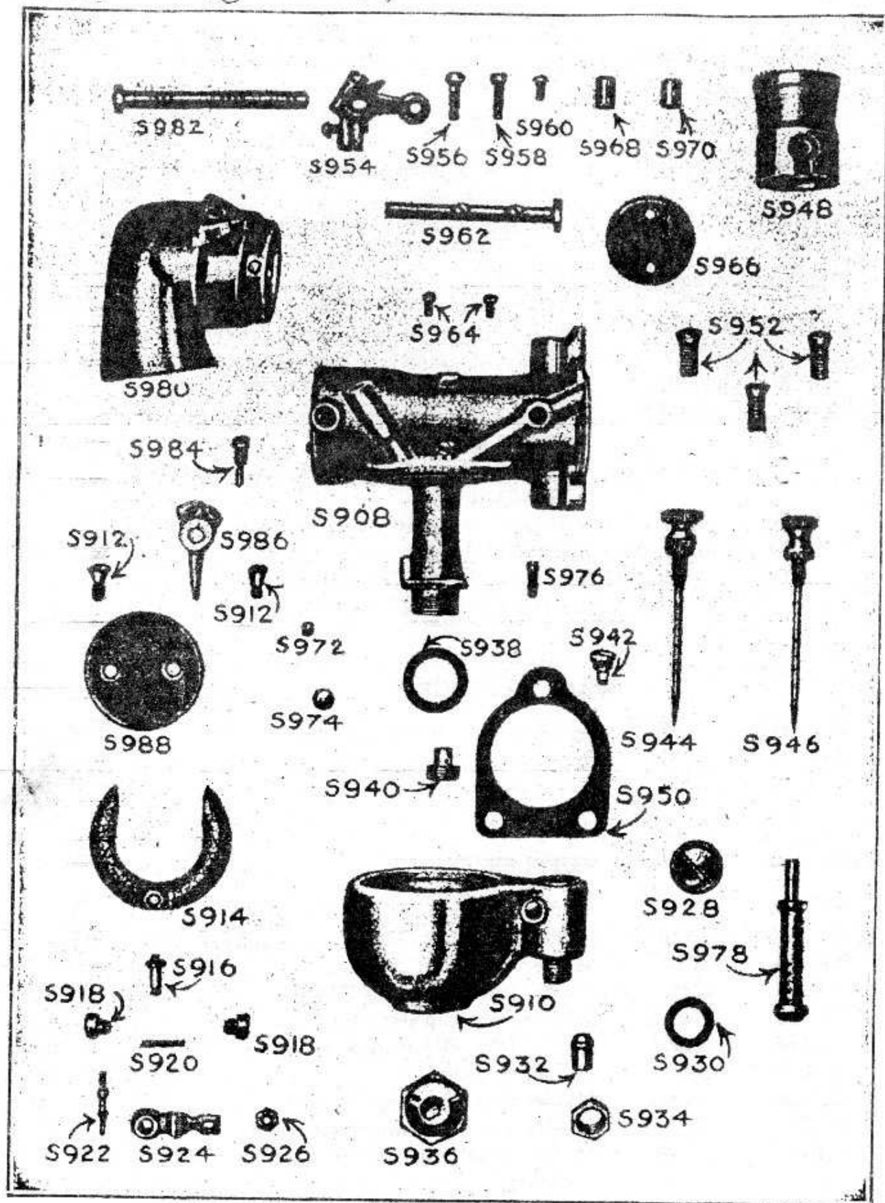
De Luxe Carburetor 1920-1927
